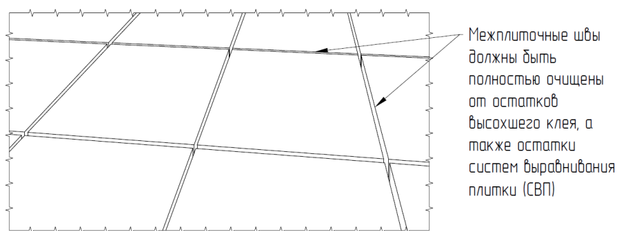
Рис. 33. Подготовка межплиточных швов
